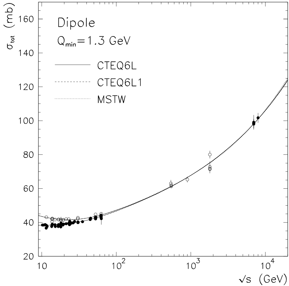
Fig. 4.3: Seção de choque total para pp (●) e \bar{p}p (○).
