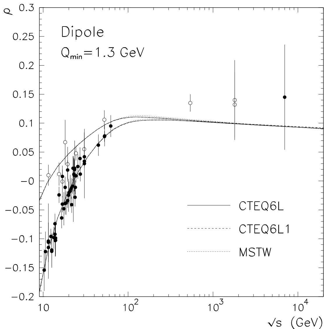
Fig. 4.5: Razão entre a parte real e imaginária da amplitude de espalhamento frontal para pp ( \bullet ) e \bar{p}p ( \circ ).
